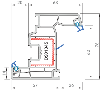
7627E Damlalıklı Kanat
