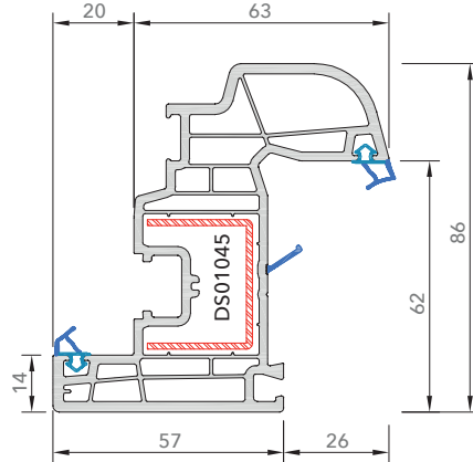
7633E Orta Contalı Orta Kayıt
