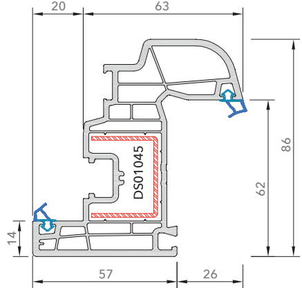
7638E Orta Contasız Orta Kayıt
