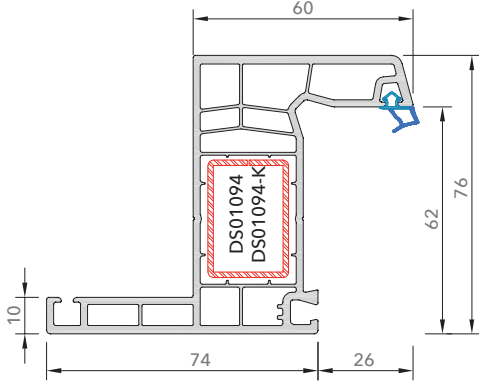
7616AE Pervazlı Kasa
