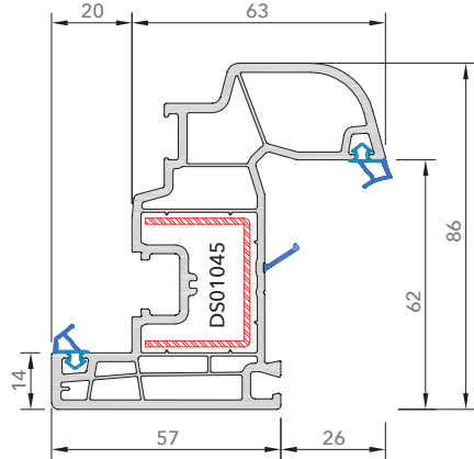
7632E Orta Contalı Orta Kayıt
