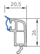
7655 - Üçlü Cam Çıtası - 40mm
