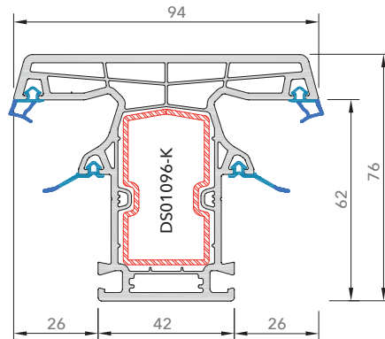
7633E Orta Contalı Orta Kayıt
