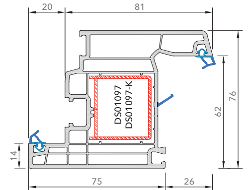
7641AE Balkon Kapı Kanat
