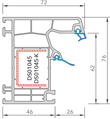
7607E Orta Contalı Pervazlı Kasa
