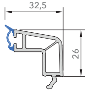
7653 - Çift Cam Çıtası - 28mm
