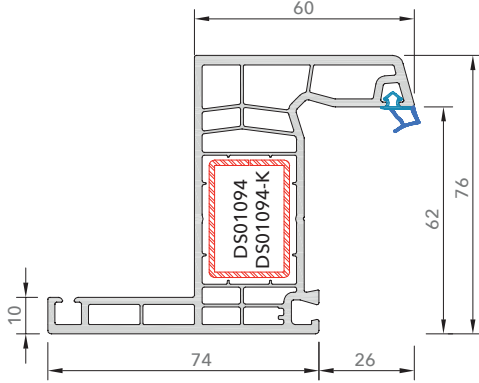
7617E Pervazlı Kasa
