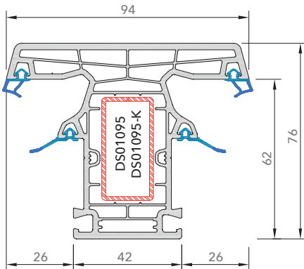
7632E Orta Contalı Orta Kayıt
