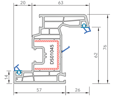
7631AE Orta Contalı Orta Kayıt
