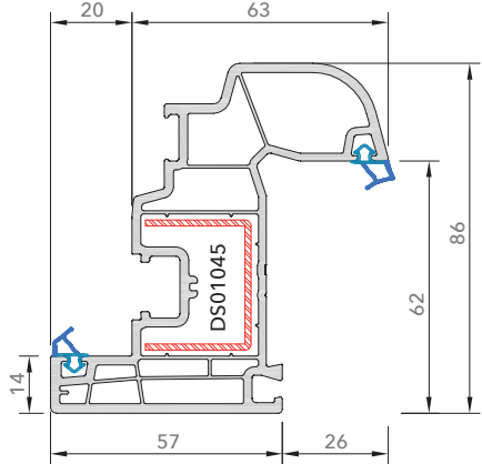
7637AE Orta Contasız Orta Kayıt
