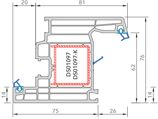
7642E Balkon Kapı Kanat
