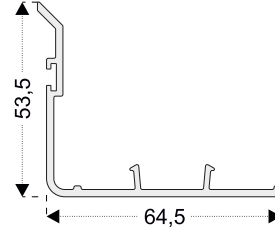
PEN25 ** PR024 için Sürme Kanat Adaptörü
