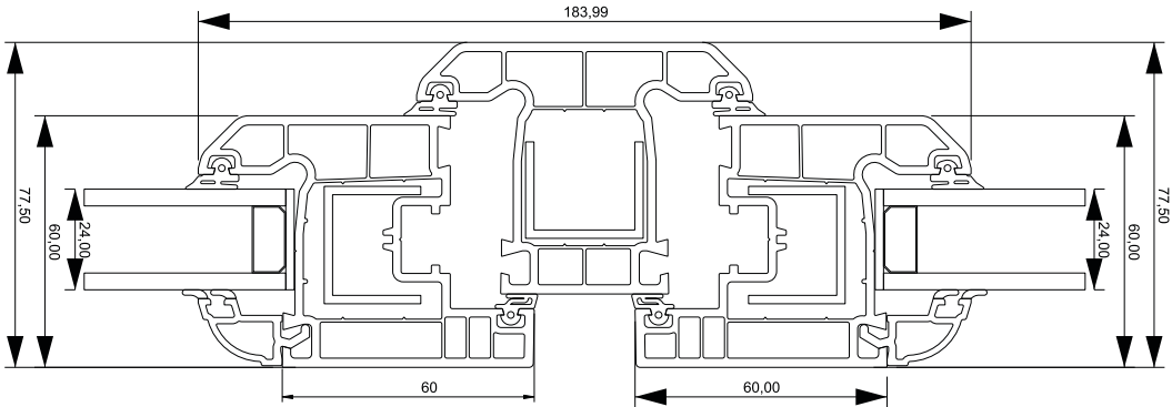
Kanat - Orta Kayıt - Kanat Kesit Detayı
