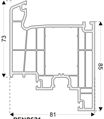
PEN8631 Z Kapı Kanat
