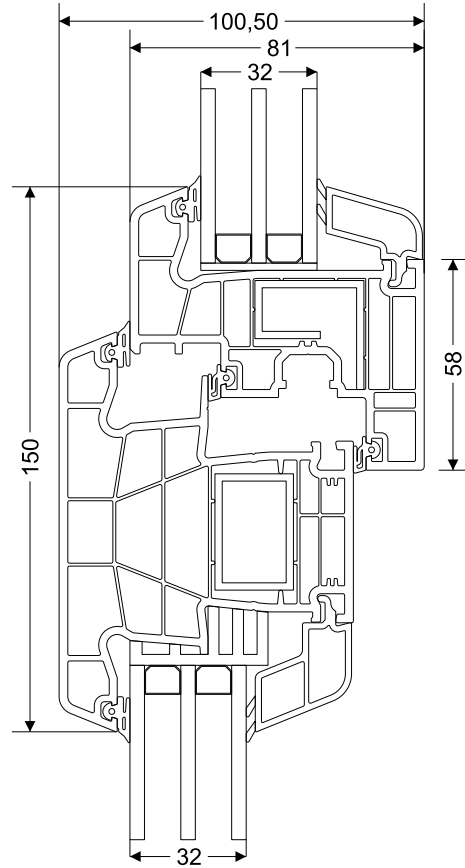
Kanat - Orta Kayıt - Sabit
