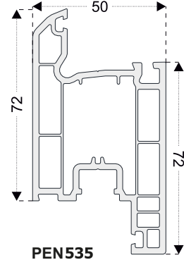
PEN535 Z Kapı Kanat
