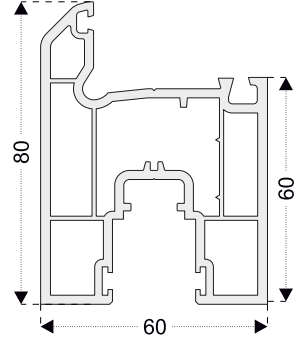
PEN21 Sürme Kanat
