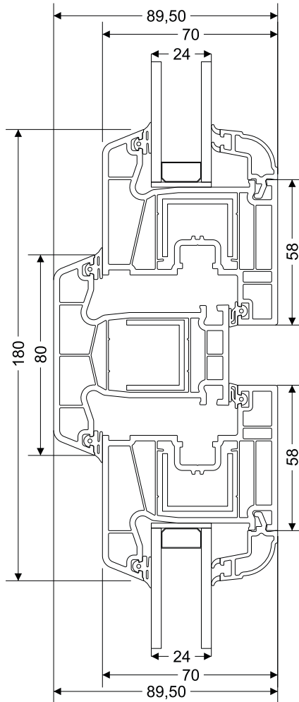
Kanat - Orta Kayıt - Kanat Kesit Detayı
