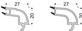
PEN701 20-22 mm Çift Cam Çita
