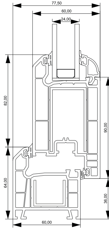
Kasa - İçe Açılan Kapı Kanat Kesit Detayı
