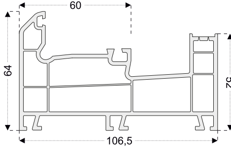
PEN23 Tek Sürme Kasa
