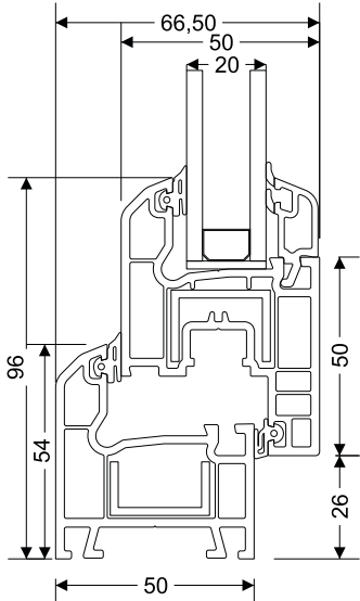
Kasa - Kanat Kesit Detayı
