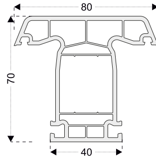
PEN713 Orta Kayıt
