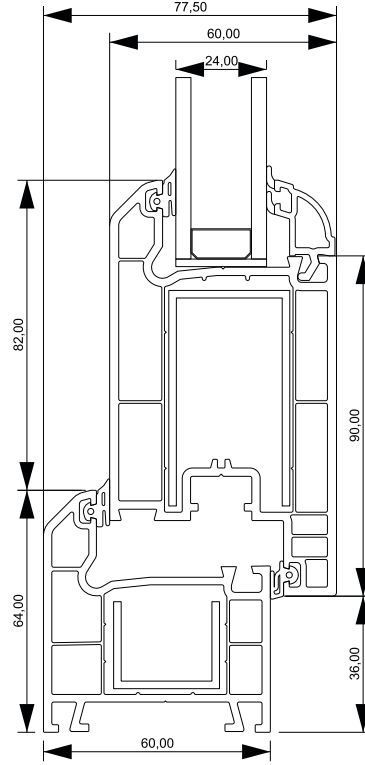
Kasa - Z Kapı Kesit Detayı
