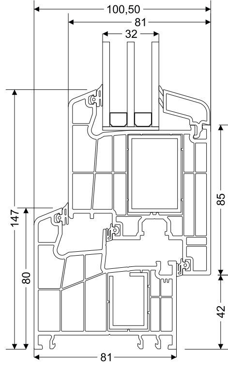
Kasa - Z Kapı Kanat Kesit Detayı
