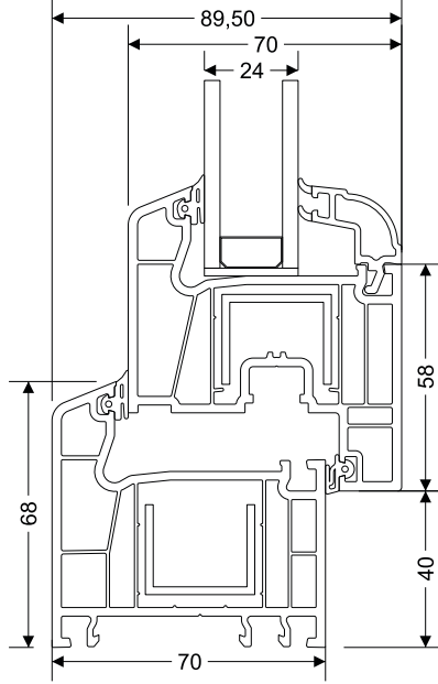
Kasa 48mm - Kanat Kesit Detayı
