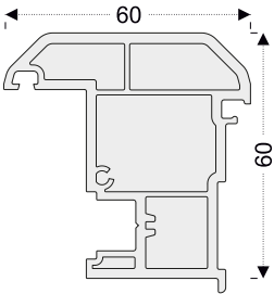
PEN12 Hareketli Orta Kayıt
