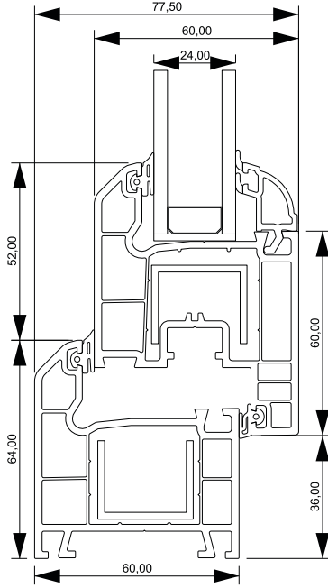
Kasa - Kanat Kesit Detayı
