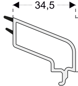
PEN8644 24mm Çift Cam Çita (Kasa, Orta Kayıt) PRO81601, PRO8621
