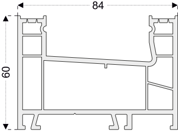
PEN20 Çift Sürme Kasa
