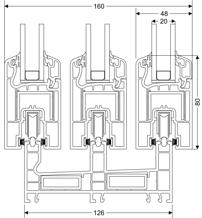
Üçlü Sürme Kasa, Kanat Kesit Detayı
