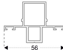
PEN41 Sürme Kanat Alın Kilitleme (Alüm.)
