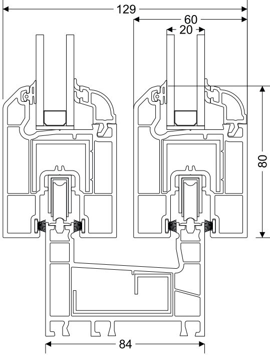
Sürme Kasa - Sürme Kanat Kesit Detayı
