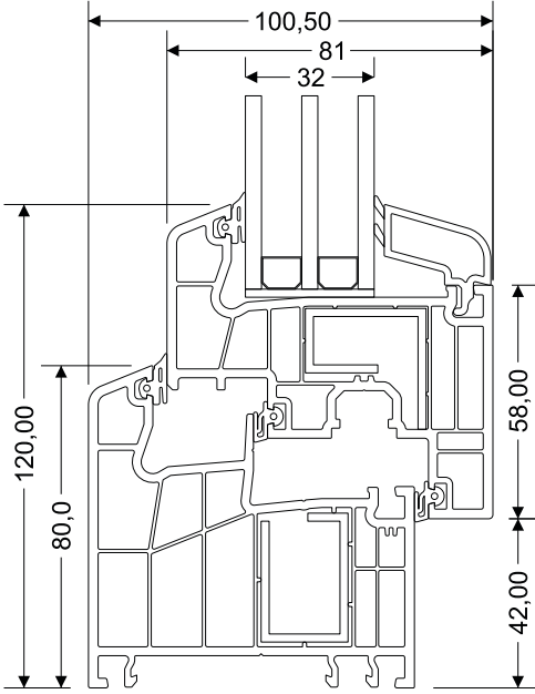
Kasa - Kanat Kesit Detayı
