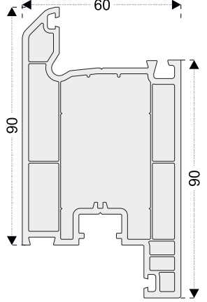
PEN04 Z Kapı Kanat
