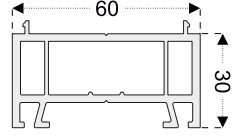
PEN 14 Yükseltme - 30mm (60mm Seri)
