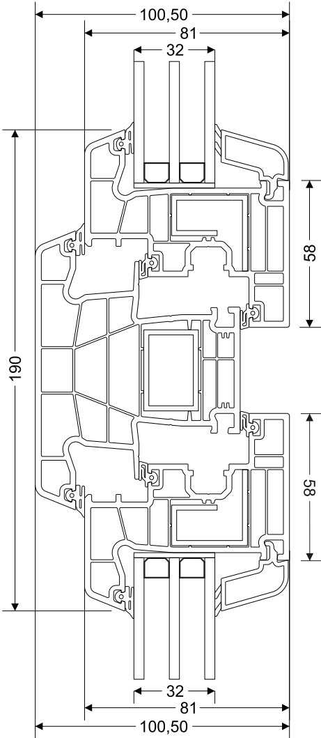
Kanat - Orta Kayıt - Kanat
