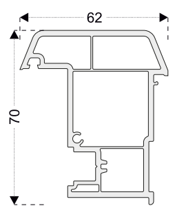
PEN717 Hareketli Orta Kayıt
