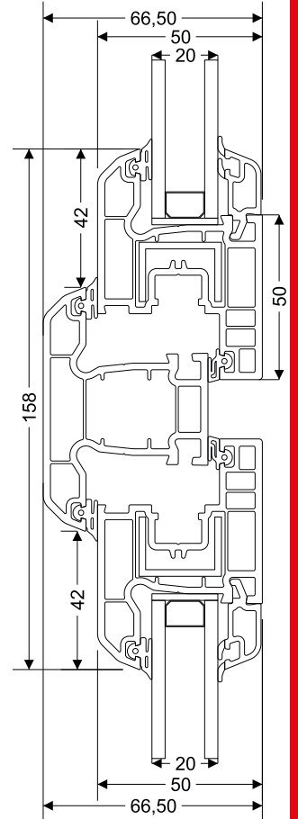
Kanat - Orta Kayıt - Kanat Kesit Detayı
