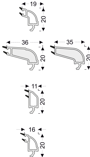
PEN05 20-22 mm Çift Cam Çita
