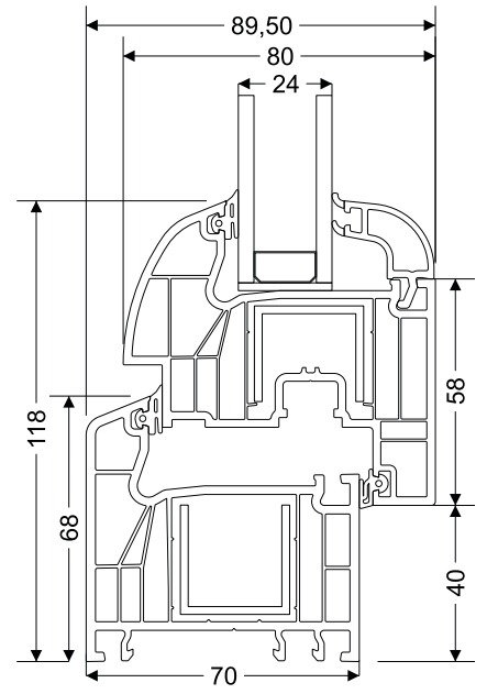
PRO7006 Kasa (6 Odacıklı) - Damlalıklı Kanat Kesit Detayı
