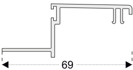
PEN28 Çift Sürme Kasa Kapama (Alüm.)
