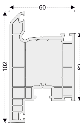
PEN10 T Kapı Kanat
