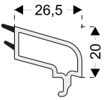
PEN8641 32mm Üçlü Cam Çita (Z Kanat, Z Kapı Kanat) PRO8611, PRO8631
