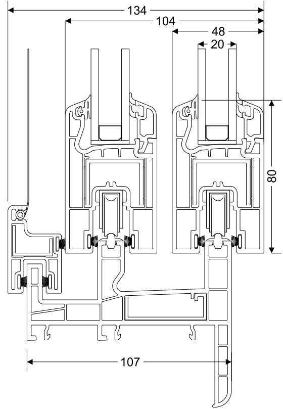
Pervazlı, Sineklikli Çift Sürme Kasa - Sürme Kanat - Sürme Sineklik Kanat Kesit Detayı
