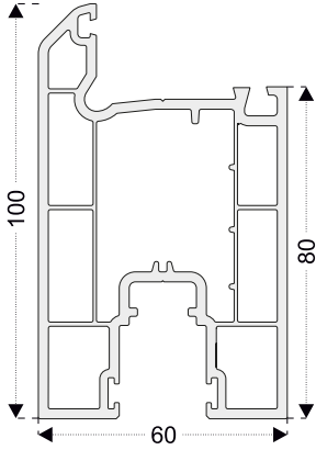
PEN24 Sürme Kanat
