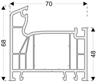
PEN720 Kasa (6 Odacıklı)
