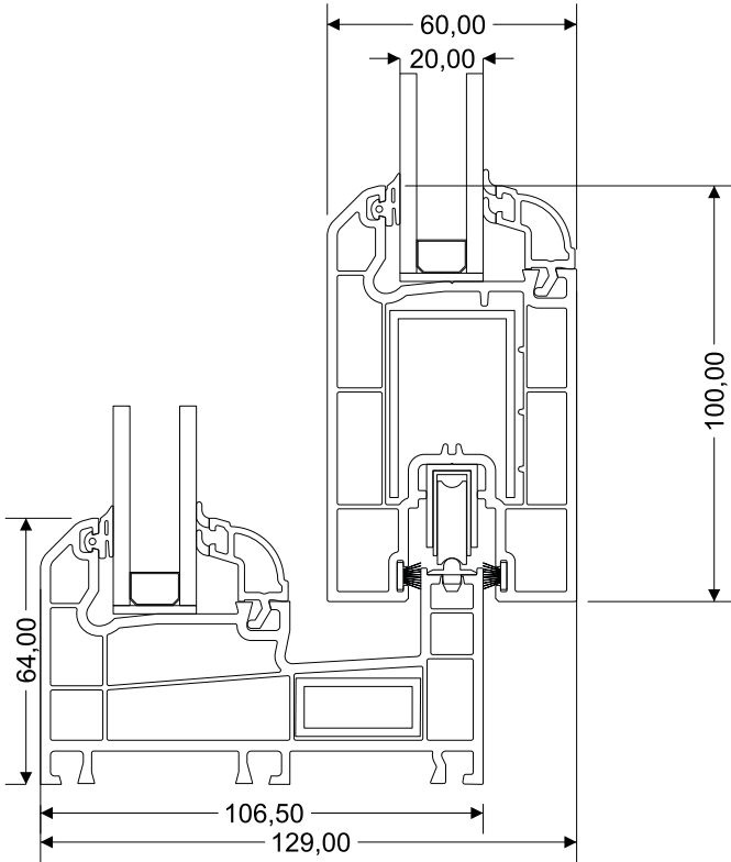
Tek Sürme Kasa, Sürme Kanat Kesit Detayı
