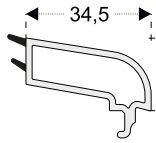
PEN8642 24mm Çift Cam Çita (Z Kanat, Z Kapı Kanat) PRO8611, PRO8631
