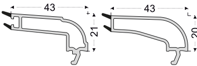
PEN700 4-6 mm Tek Cam Çita
