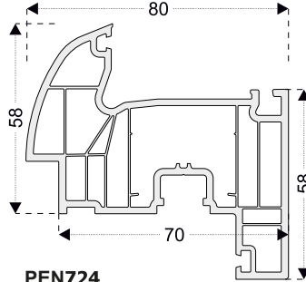
PEN724 Damlalıklı Kanat (7 Odacıklı)
