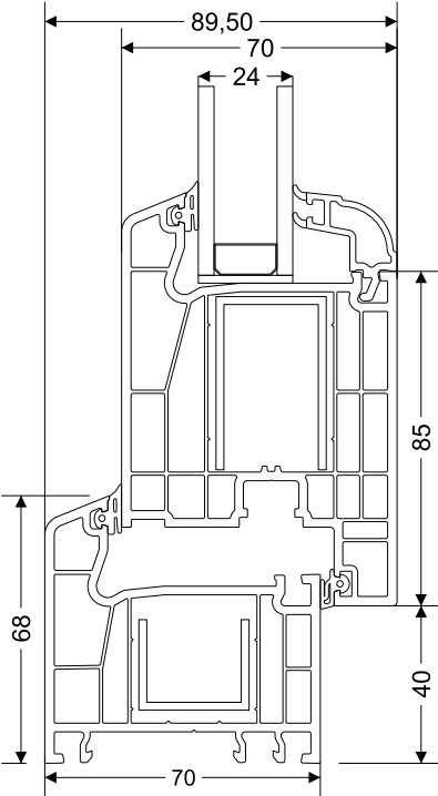
Kasa - Z Kapı Kanat Kesit Detayı
