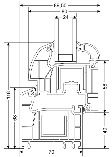
Kasa - Damlalıklı Kanat Kesit Detayı
