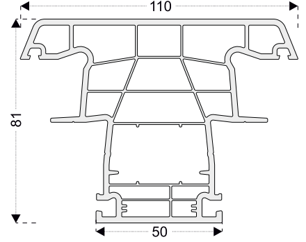
PEN8621 Orta Kayıt
