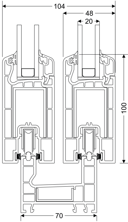
Sürme Kasa - Sürme Kanat Kesit Detayı
