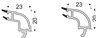
PEN702 24-26 mm Çift Cam Çita
