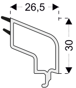
PEN8643 32mm Üçlü Cam Çita (Kasa, Orta Kayıt) PRO8601, PRO8621
