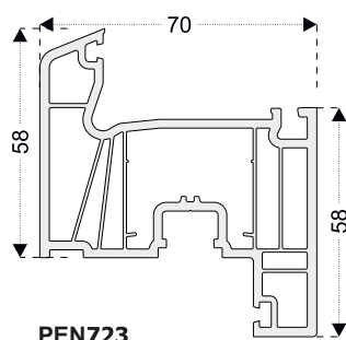
PEN723 Kanat (6 Odacıklı)
