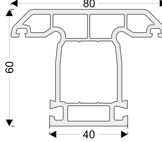
PEN53 Orta Kayıt
