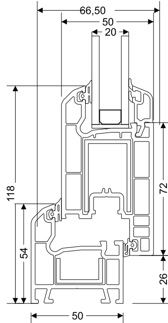
Kasa - Z Kapı Kanat Kesit Detayı
