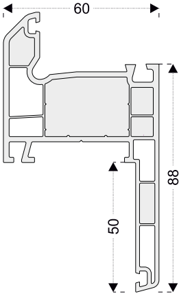
PEN82 Pervazlı Kasa
