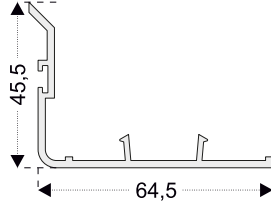
PEN22 ** PR021 için Sürme Kanat Adaptörü
