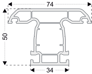
PEN533 Orta Kayıt
