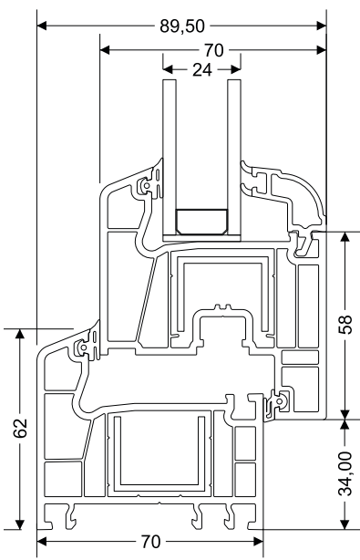
Kasa 42mm - Kanat Kesit Detayı
