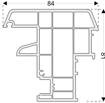
PEN8622 Hareketli Orta Kayıt
