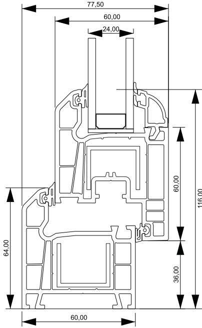
Kasa-Kanat Kesit Detayı
