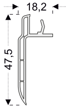
PEN 38 Tırnaklı Pervaz (60mm Seri)
