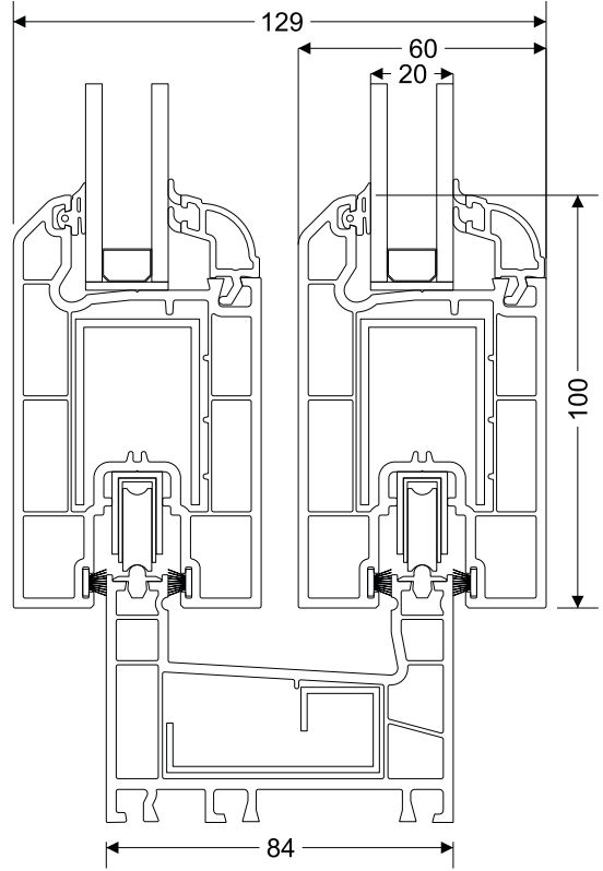
Sürme Kasa - Sürme Kanat Kesit Detayı
