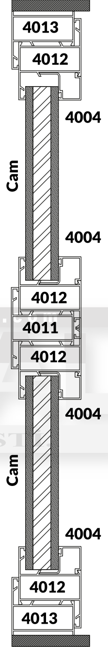
Dar Kasa Isı Cam Aldoks Montaj Kesiti
