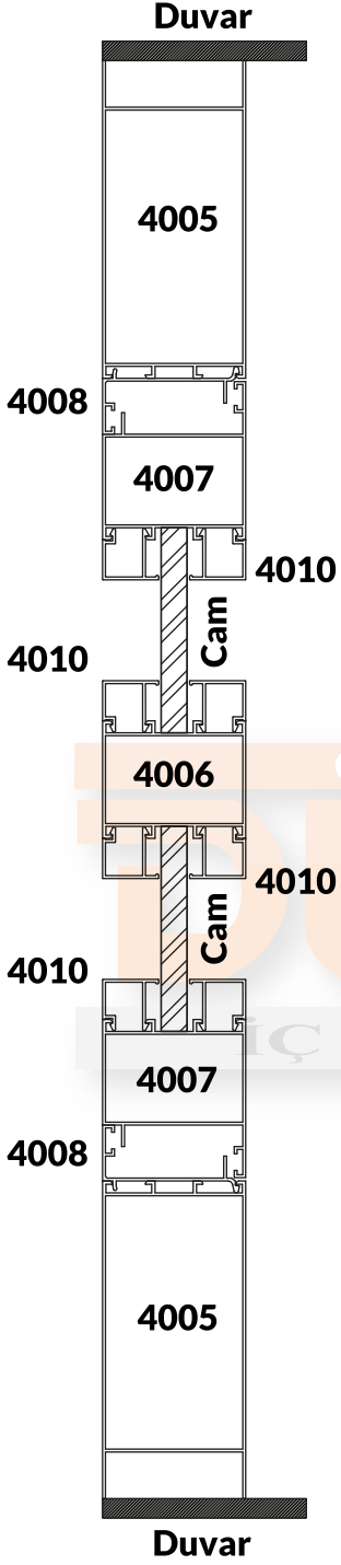
Etek Profilli Tek Cam C60 Montaj Kesiti
