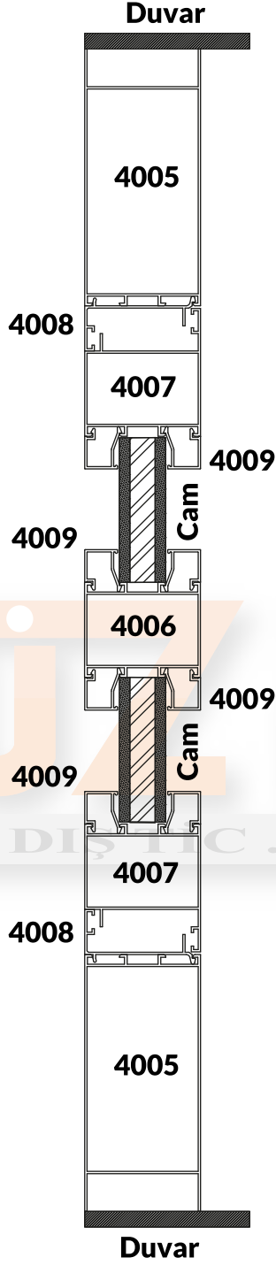
Etek Profilli Isı Cam C60 Montaj Kesiti
