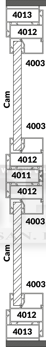
Dar Kasa Tek Cam Aldoks Montaj Kesiti
