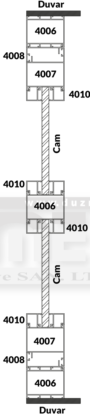
Kasa Profilli Tek Cam C60 Montaj Kesiti
