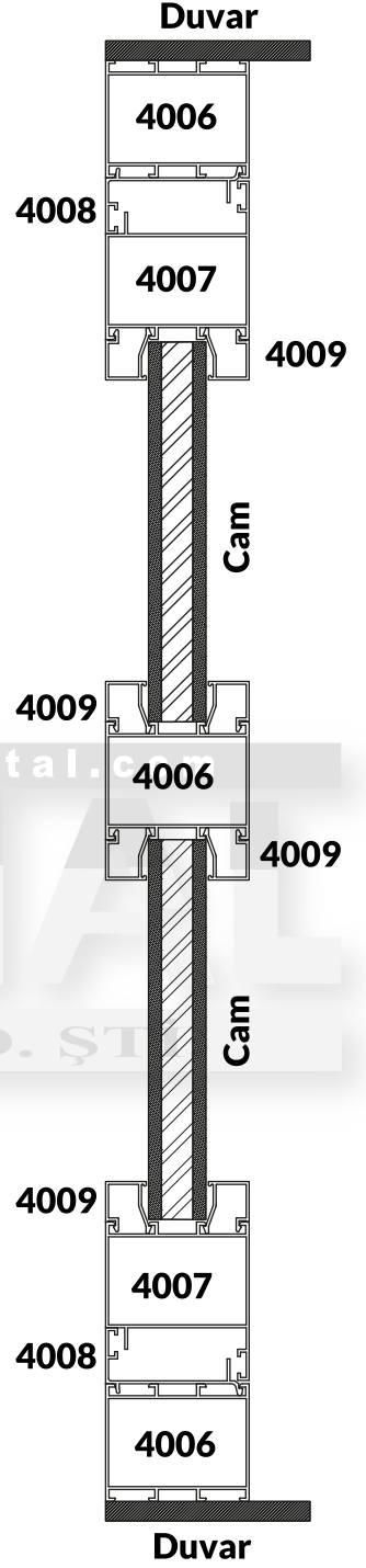
Kasa Profilli Isı Cam C60 Montaj Kesiti
