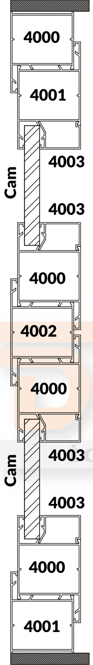
Genis Kasa Tek Cam Aldoks Montaj Kesiti
