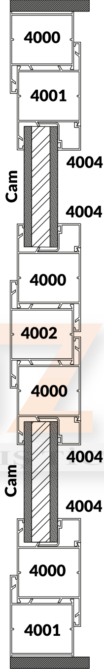
Genis Kasa Isı Cam Aldoks Montaj Kesiti
